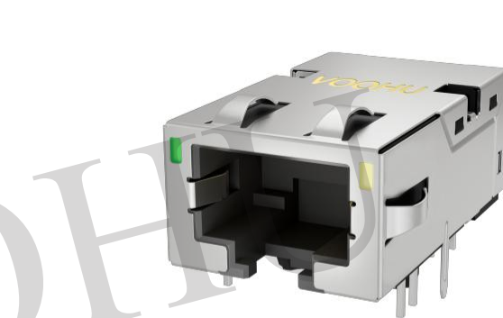
结构图:
