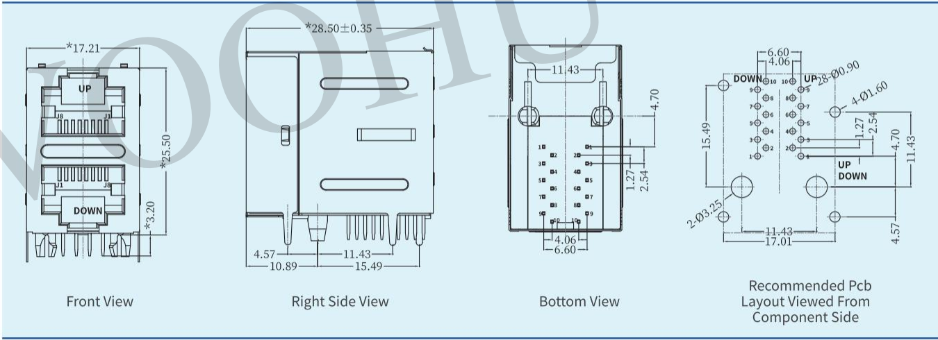
结构图:
