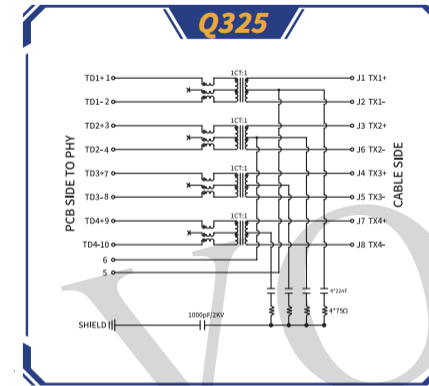
线路图 Q319-Q390
