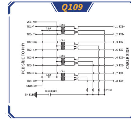
线路图 Q108-Q250
