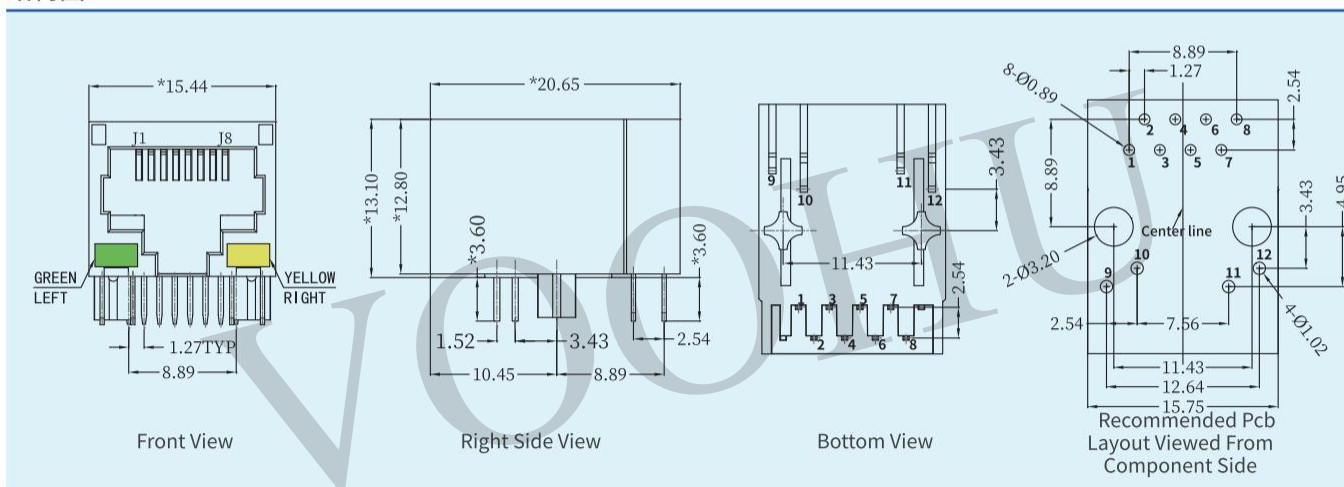
结构图：
