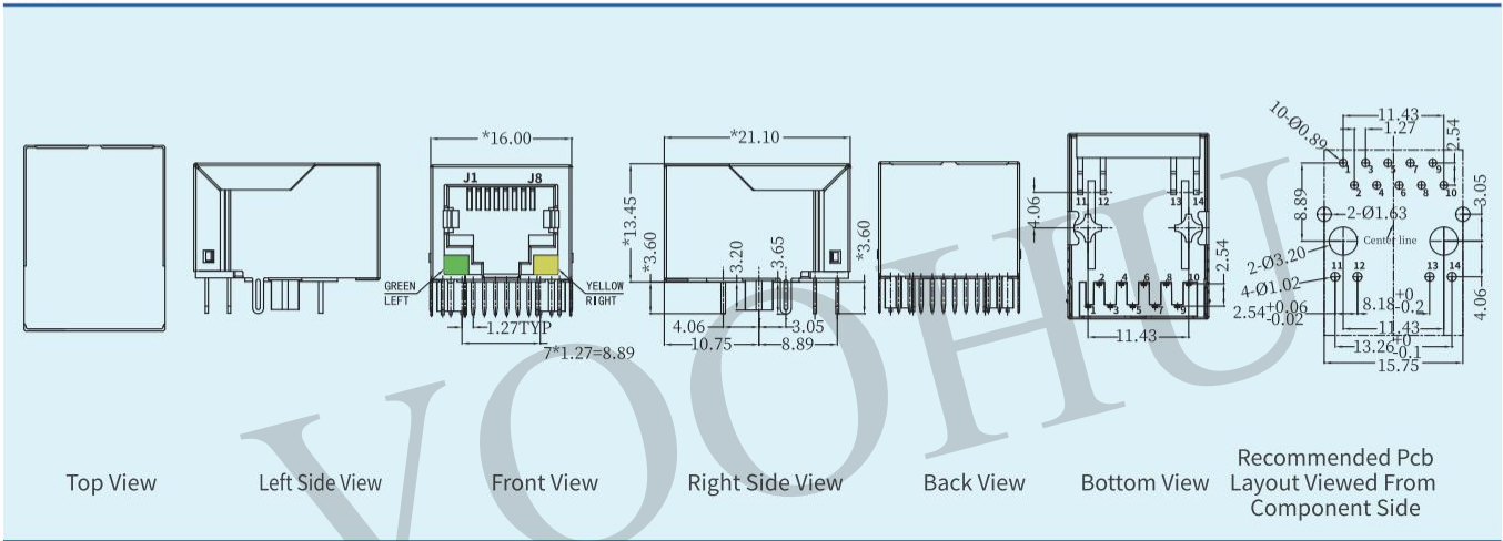
结构图:
