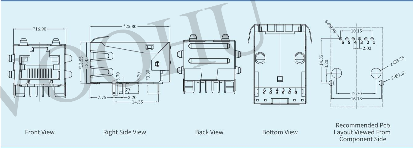
结构图:
