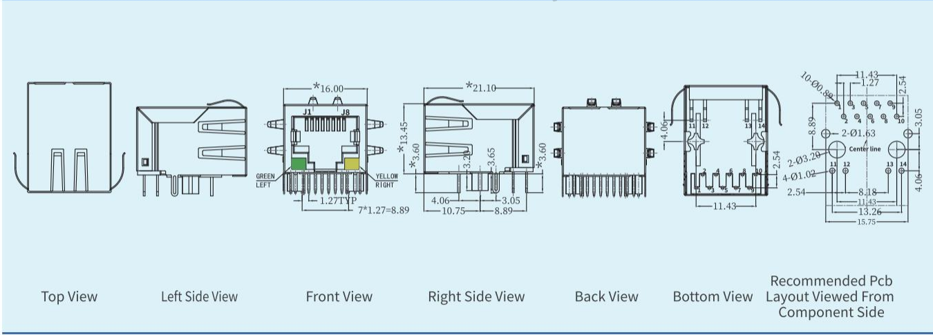
结构图:
