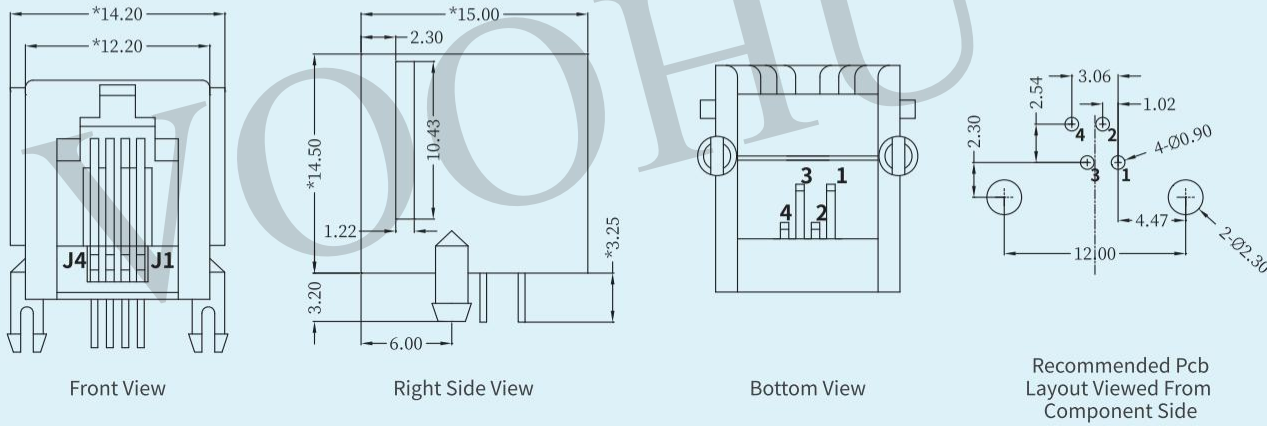
结构图:
