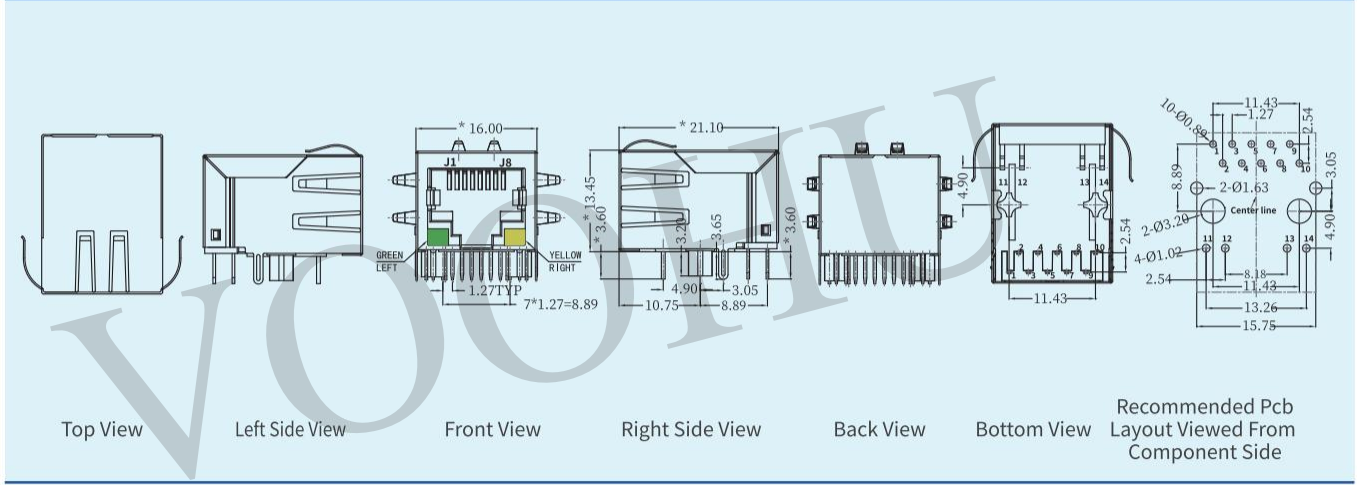
结构图:
