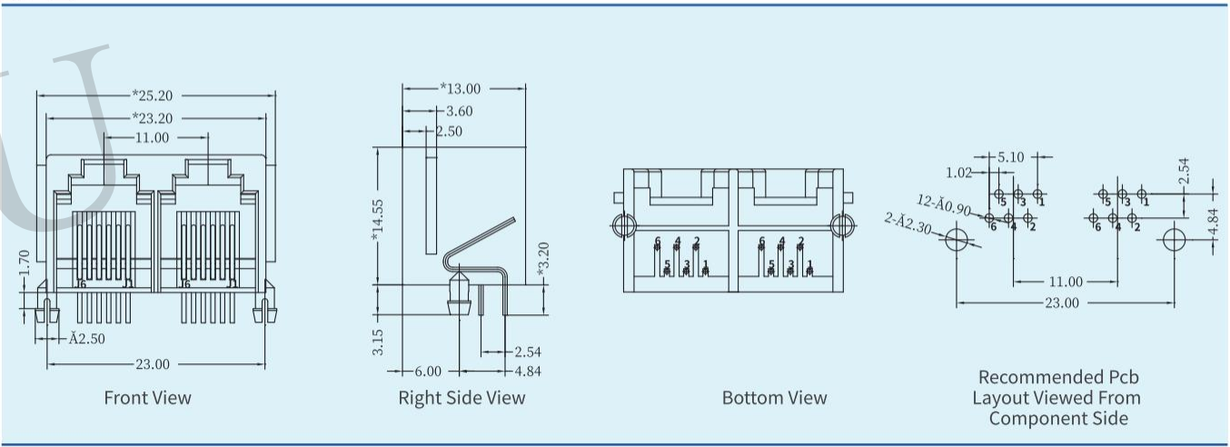
结构图:
