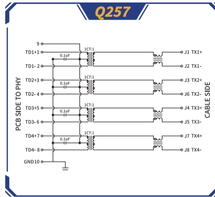
线路图 Q254-Q318
