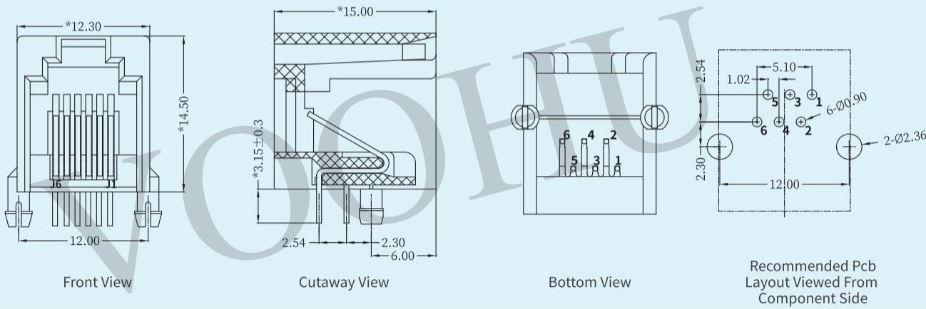
结构图:
