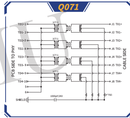
线路图 Q070-Q106
