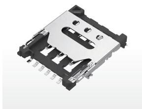
● NANO SIM翻盖式
