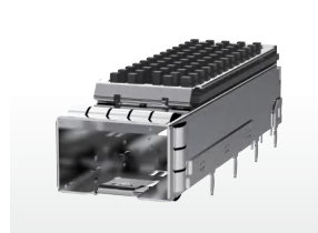
● SFP CAGE 带散热器
