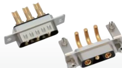
● 大电流型D-SUB
