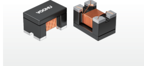
• 2012系列CMC共模电感
